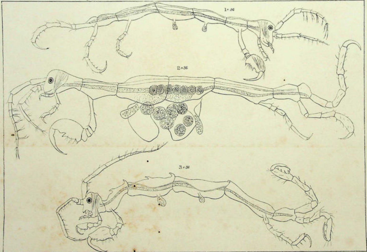
1. 2. CAPRELLA MADRASANA n. sp., ♂, ♀. 3. ——— PALKII . n. sp., ♀.
