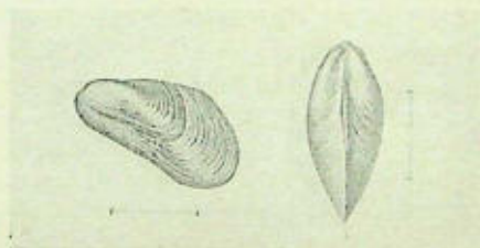
FIG. 2.— Modiola cochinensis , sp. nov., \times 2 .
