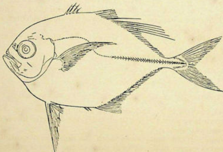
FIG. 2.— Caranx auricoronæ , sp. nov.
