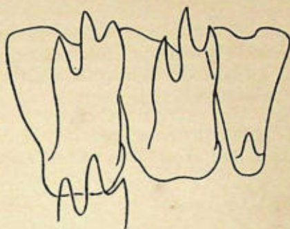
FIG. 2.—Radula of Limnæa bowelli , Preston.
