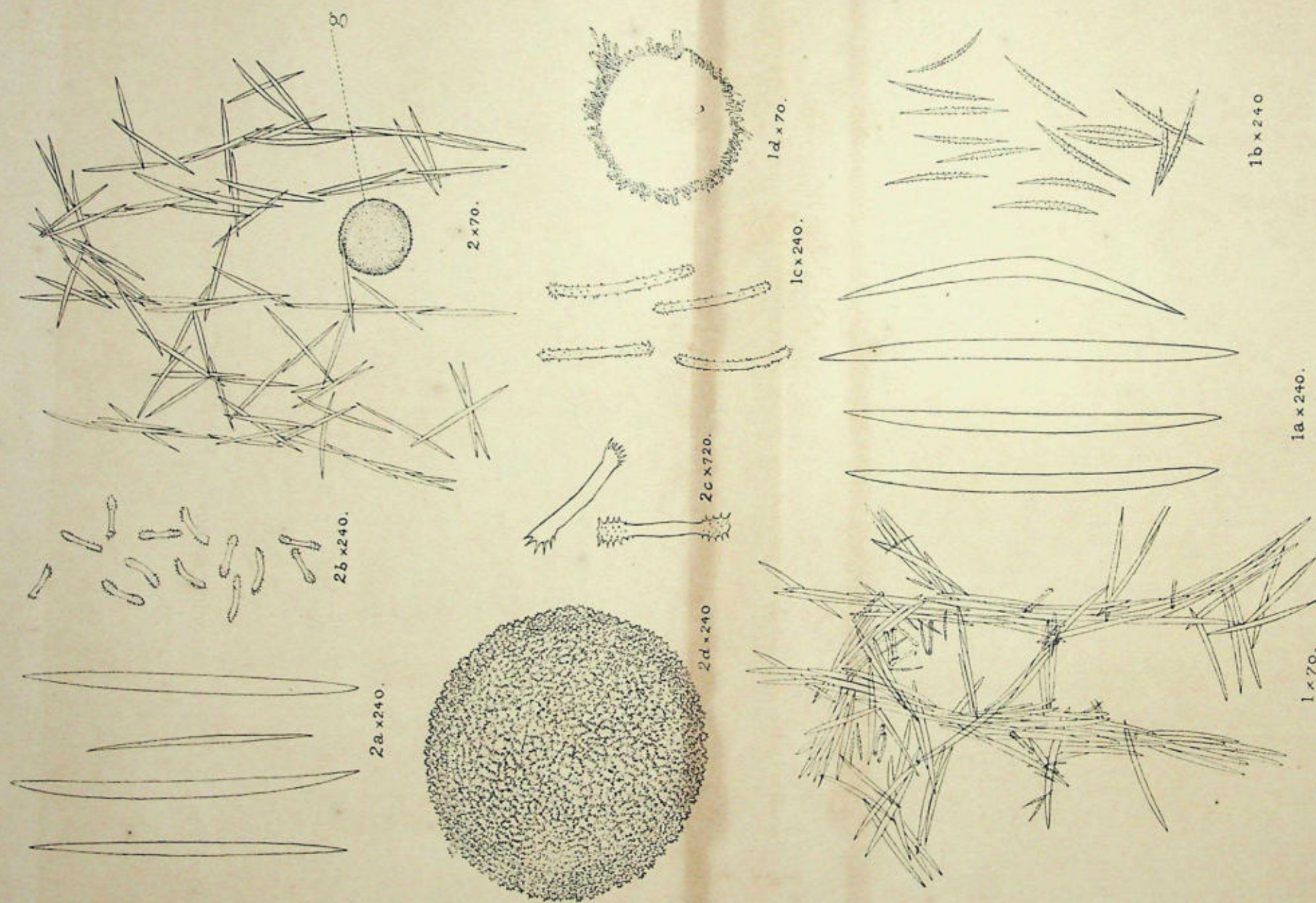
Fig.1 Spongilla travancorica sp. nov.
