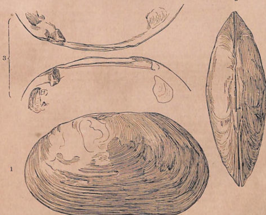
Fig. 9.—1 & 2. Pseudodon ( T. ) peguensis ( Ant. ) var. curvata , Preston. (Type.) Nat. size.
