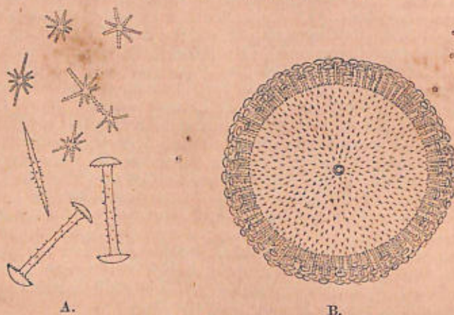
Fig. 22.— Dosilia plumosa .
