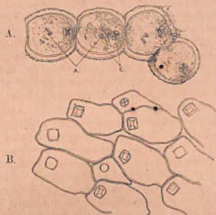
Fig. 39.— Histopia lacustris .
