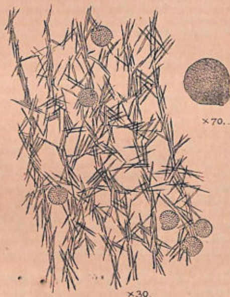
Fig. 24.— Trochospongilla latouchiana .
