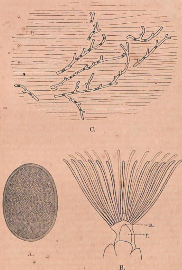
Fig. 41.— Fredericella indica .
