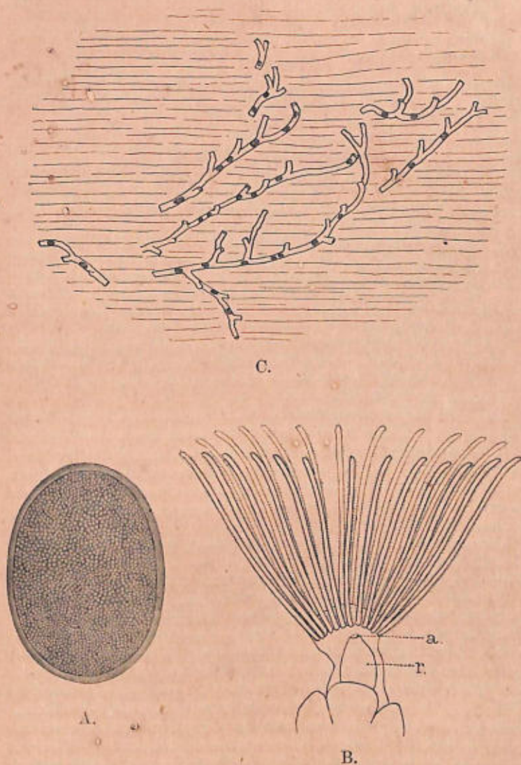
Fig. 41.— Fredericella indica .
